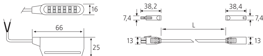
Mini-AMP-6-fach-Verteiler Distributeur sextuple Mini-AMP
